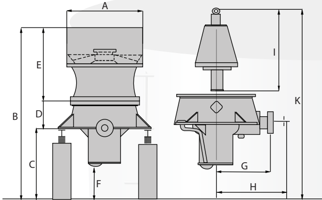
VS-Type
